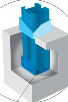
Główna konstrukcja nośna zabezpieczona do odporności ogniowej R 30
